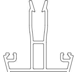
THERMAL T BAR KLP-11
